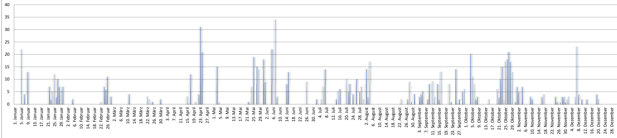
Niederschlag in mm
