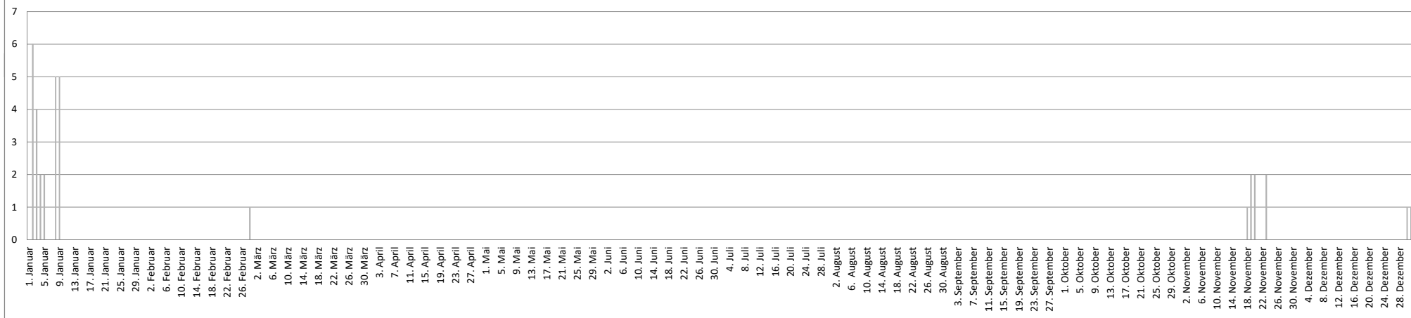
Schneefall in cm (Neuschnee)
