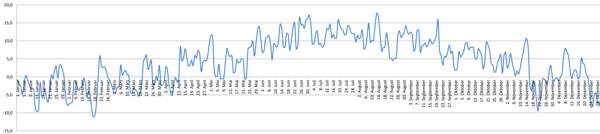
Tiefsttemperatur in der Nacht
