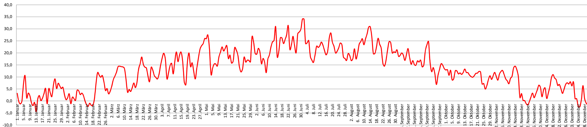
Höchsttemperatur am Tag
